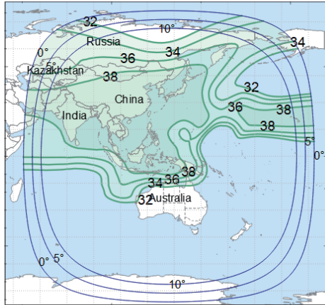
V-Pol (dBW)
