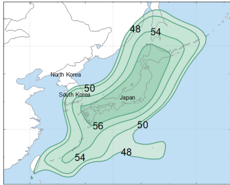
V-Pol (dBW)
