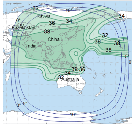
H-Pol (dBW)
