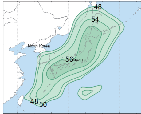
H-Pol (dBW)
