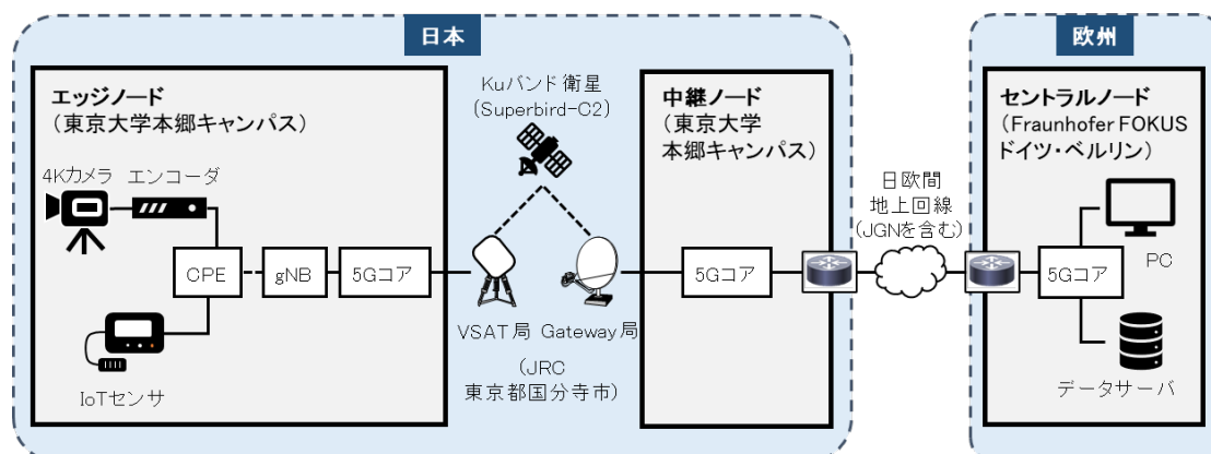
図 1 : 日欧共同実験で構築したテストベッドの構成
