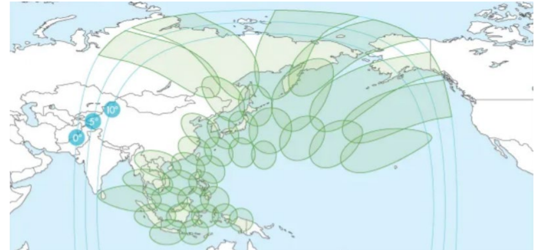
JCSAT-1C が搭載する Ku 帯スポットビームのカバーエリア
