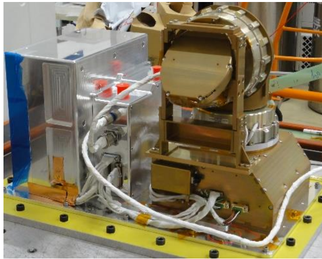
図 1 : 光通信装置の外観写真【Credit: 情報通信研究機構 (NICT)・ソニーコンピュータサイエンス研究所 (Sony CSL)・次世代宇宙システム技術研究組合 (NeSTRA)】
