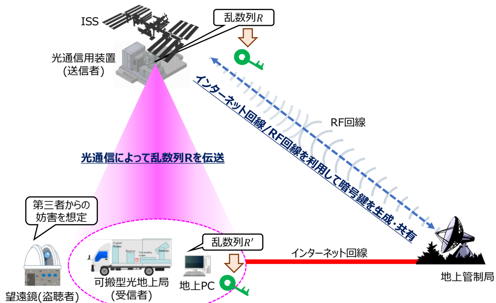
図 2 : ISS-地上間での実証実験イメージ【Credit: 情報通信研究機構 (NICT)・スカパーJSAT】
