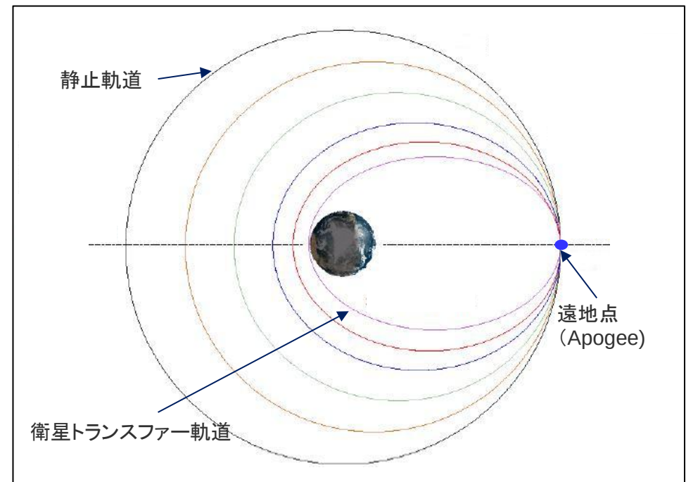
衛星トランスファー軌道
