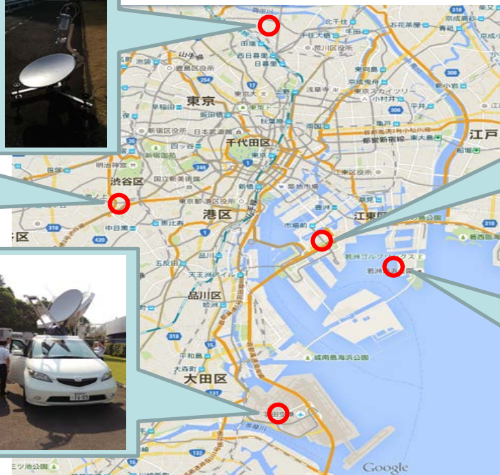
■ 東京女子医科大東医療センター 手動捕捉型可搬局 (日本アンテナ様)
